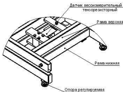
Рис.2 Пример крепления датчика в весах (в зависимости от конструктивного исполнения может отличаться)
